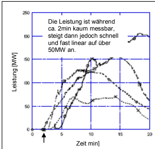
Abb. 15: Zeitliche Entwicklung der Brandleistung
