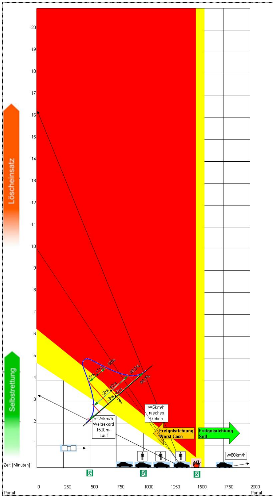
Abb. III.3 Beispiel Raum-Zeit-Diagramm
