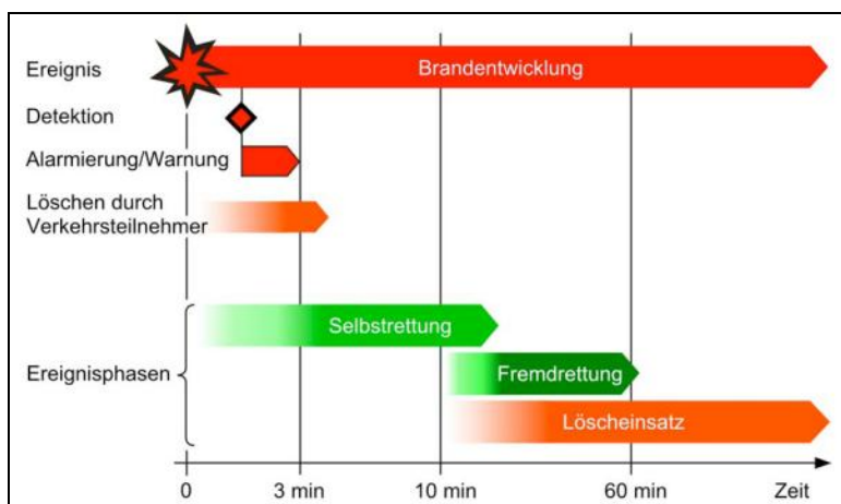
Abb. 5: Ereignisphasen bei Tunnelbrand
