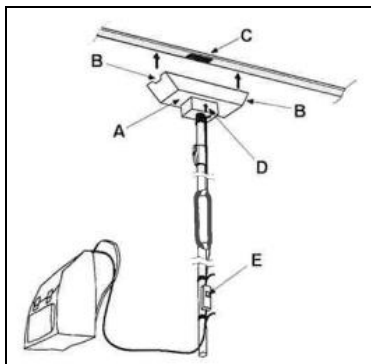
Abb. 18: Testeinrichtung für ein Brandmeldekabel (Securiton)
